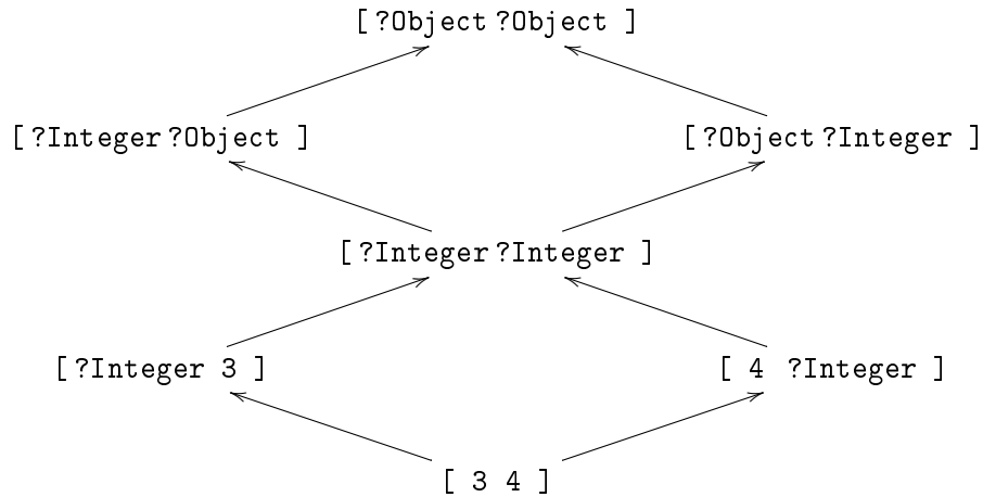
FIGURE 1 – Ordre partiel de la propriété de correspondance
