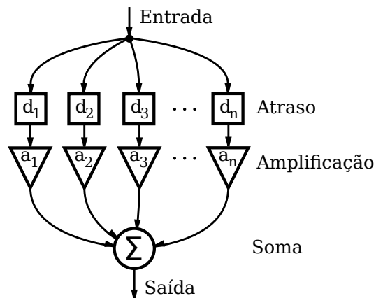
Figura 2.1: Exemplo esquemático de um filtro FIR ou de resposta ao impulso finita. Esse tipo de filtro digital é caracterizado por uma resposta ao impulso que se torna nula após um tempo finito.
