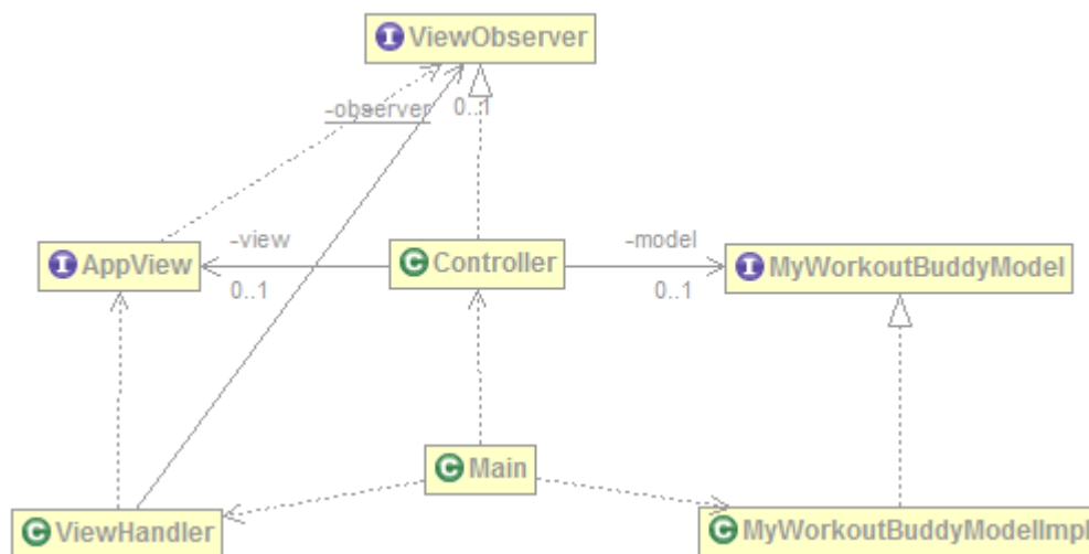
Figura 2: Schema architeturale dell'applicazione. In questo software, un Controller è un osservatore di AppViews ed è responsabile anche di gestire le interazioni con MyWorkoutBuddyModel. Si fa presente che MyWorkoutBuddyModel è l'entry-point del modello e non il modello completo. Lo stesso discorso vale per AppViews, in quanto non è altro che l'entry-point della logica di presentazione. Main è il componente responsabile di creare ogni istanza di model, view e controller e di connetterli correttamente tra loro.
