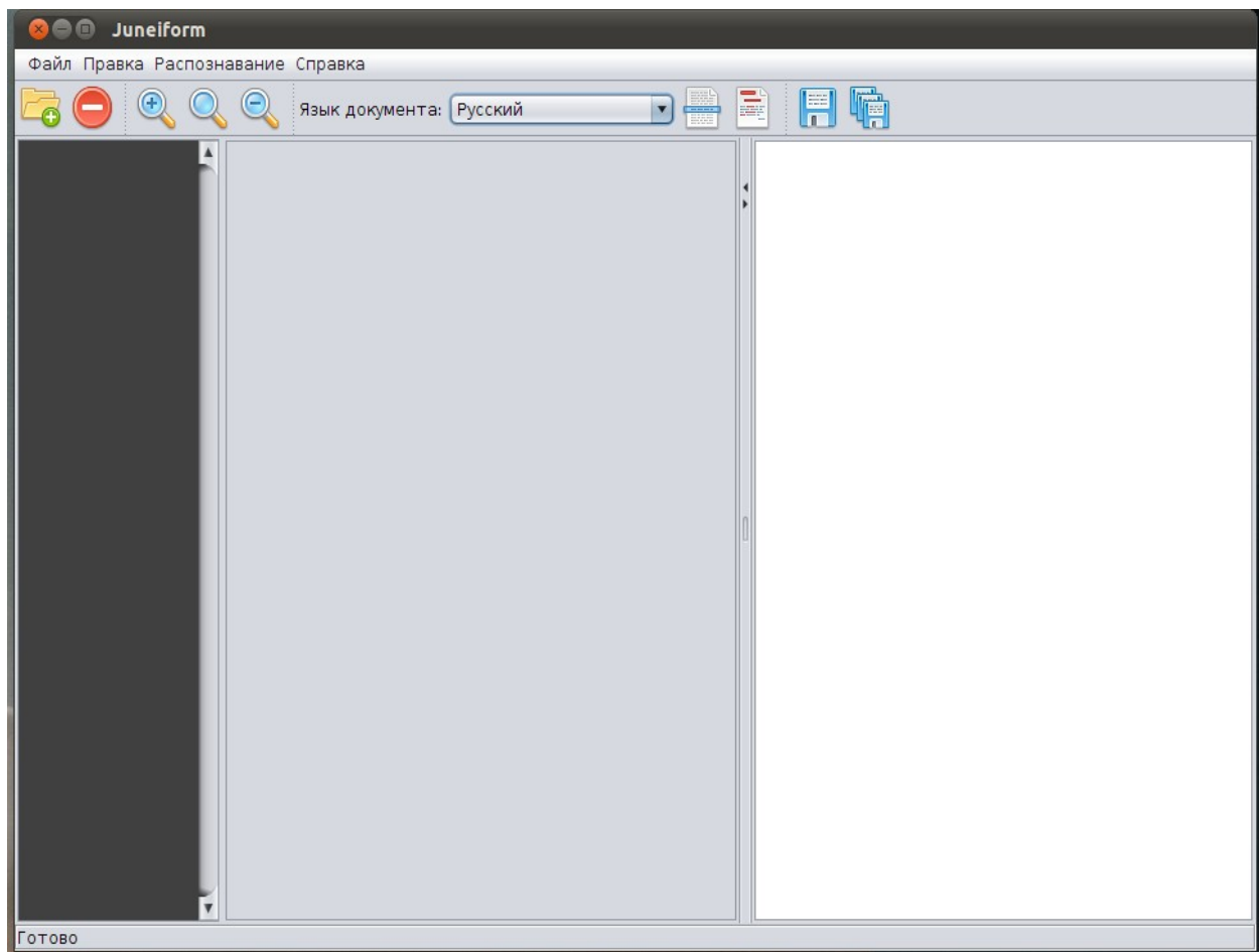
Интерфейс Juneiform.
